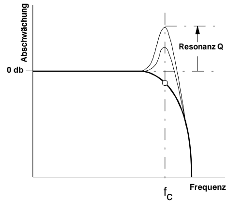
Abb. 2: Einfluß der Resonanz auf das Durchlaßverhalten beim Tiefpaß-Filter
